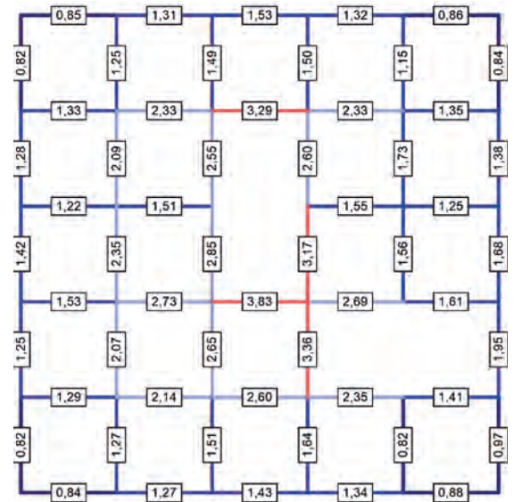
Abb. 41: Eigene Darstellung, PTV Visum, Stochastische Umlegung
