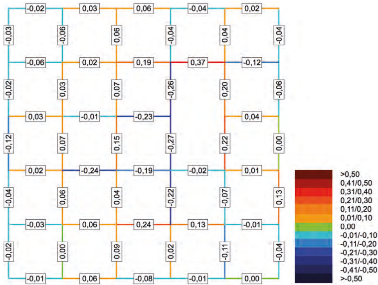
Abb. 38: Eigene Darstellung, Differenz PTV Visum - depthmapX
