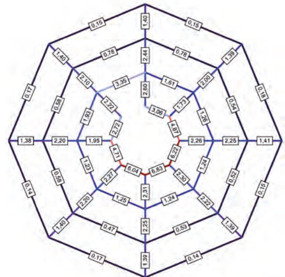
Abb. 53: Eigene Darstellung, PTV Visum, Stochastische Umlegung
