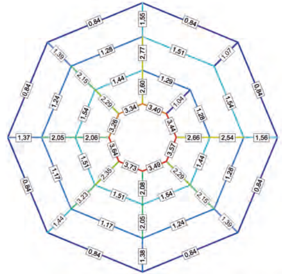
Abb. 48: Eigene Darstellung, depthmapX, Segment Map, Metric Choice
