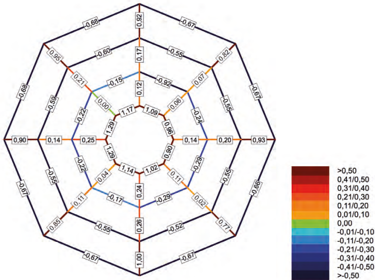
Abb. 46: Eigene Darstellung, Differenz PTV Visum - depthmapX
