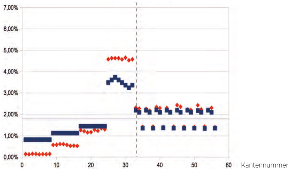
Abb. 47: Eigene Darstellung, Gegenüberstellung der Kantenwerte, blau depthmapX - rot PTV Visum
