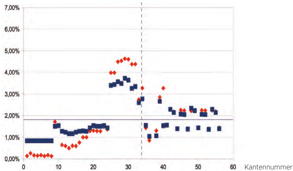
Abb. 51: Eigene Darstellung, Gegenüberstellung der Kantenwerte, blau depthmapX - rot PTV Visum
